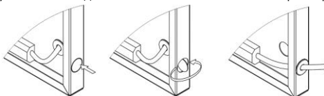
Рисунок 6 — Вывод кабеля с торца светильника.
