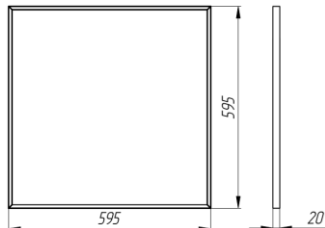
Рисунок 1 – Габаритные размеры светильника Офис 595x595x20.
