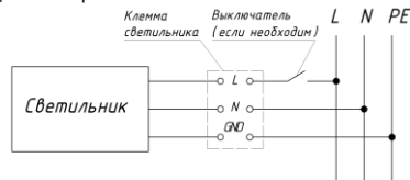
Рисунок — Схема подключения светильника.
