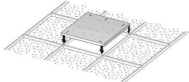
Рисунок 4 — Установка светильника Geniled серии Офис в подвесной потолок.
