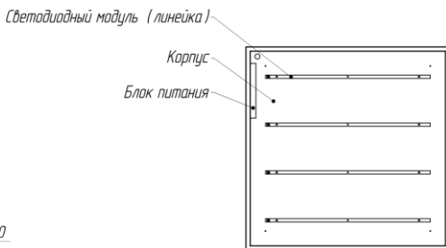
Рисунок 1 – Габаритные размеры светильника ЛПО 1200x180x20. Рисунок 2 – Состав светильника Geniled Офис
